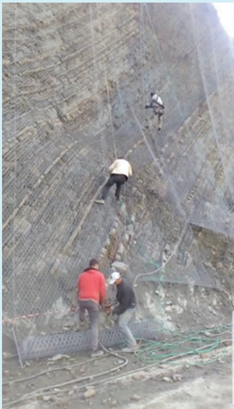
Συρματοκουρτίνα στο φυσικό πρανές και πάκτωση στη βάση με ειδικά αγκύρια. ΣΩΣΤΗ ΔΟΥΛΕΙΑ!
